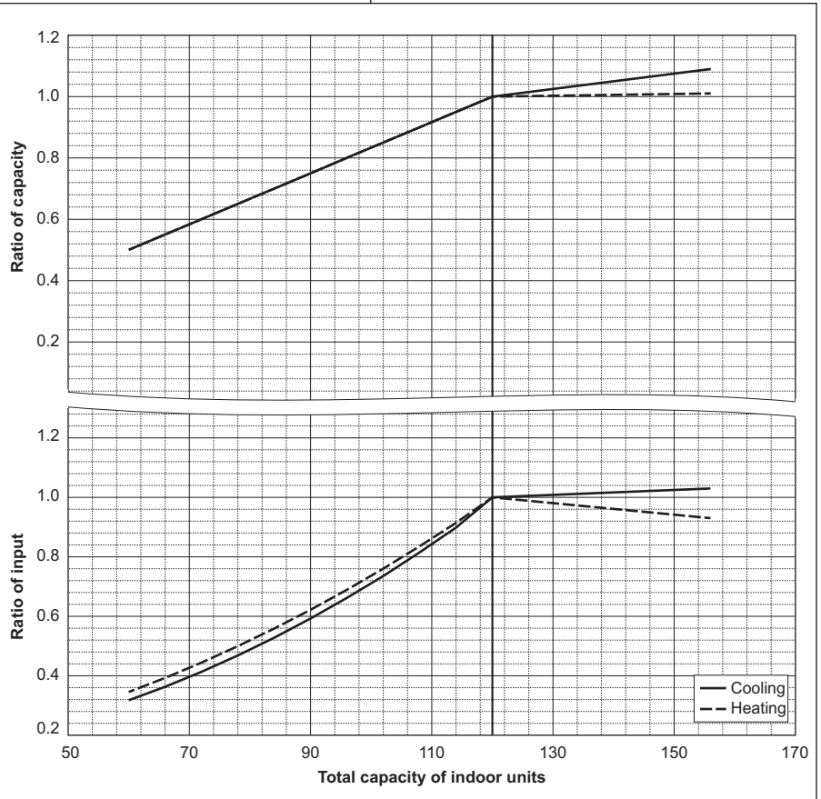
PUHY-HP144TSNU/YSNU-A
