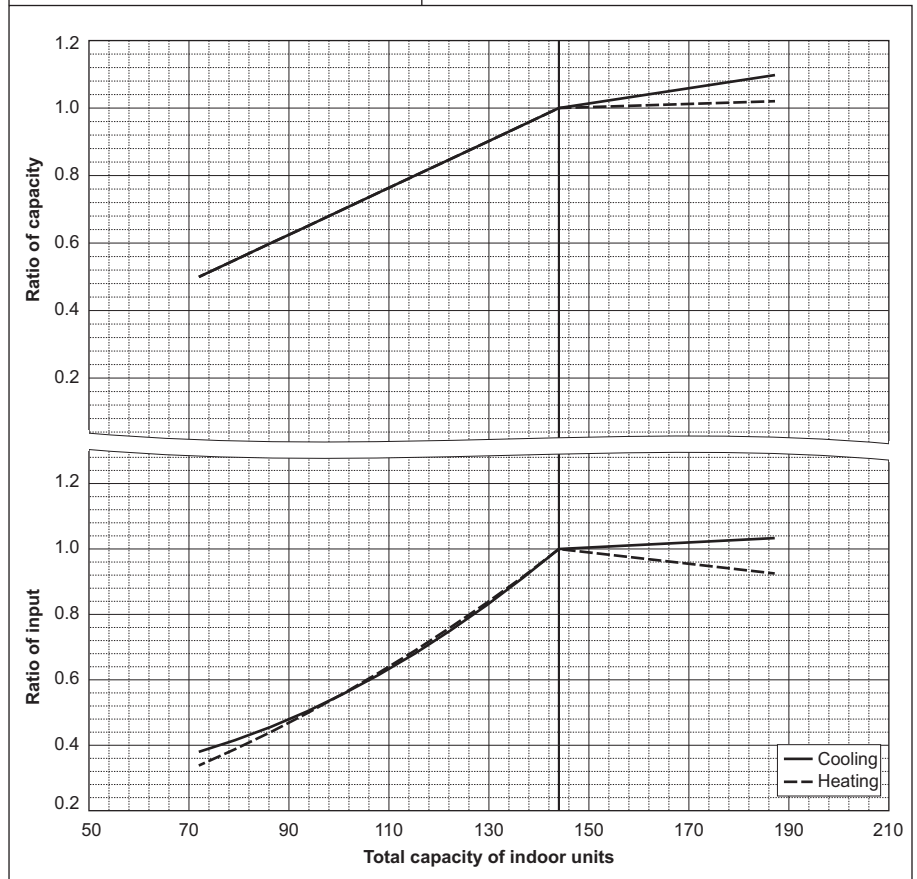
PUHY-HP144TSNU/YSNU-A
