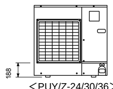
<PUY/Z-24/30/36>
