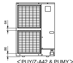
<PUY/Z-A42 & PUMY>
