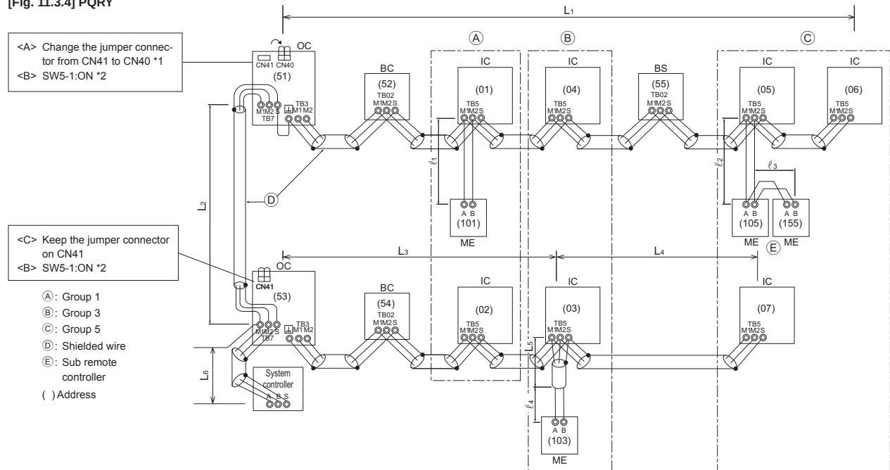
[Fig. 11.3.4] PQRY
