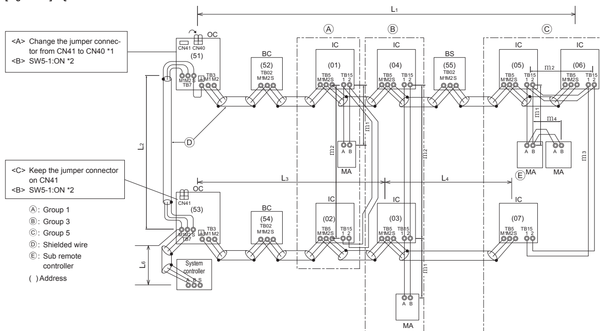
[Fig. 11.3.5] PQRY
