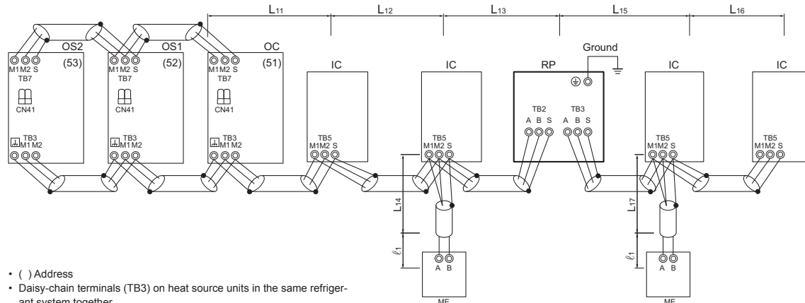
[Fig. 11.3.3] PQHY
