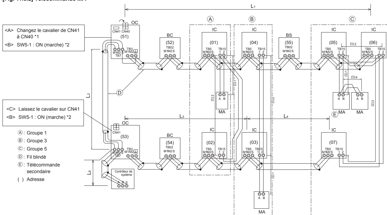
[Fig. 11.3.2] Télécommande MA
