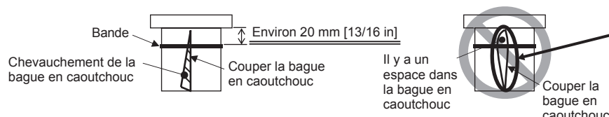
<Fig. 6: Partie arrière de la bague en caoutchouc>
