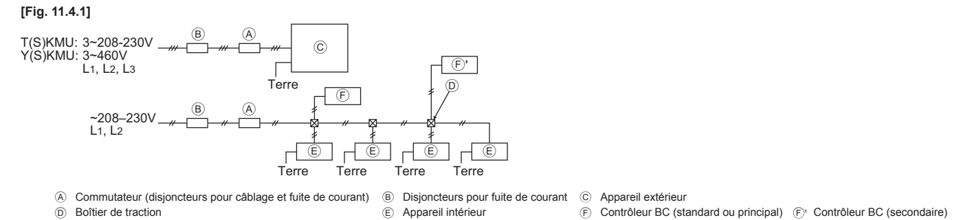
Épaisseur de câbles pour l'alimentation électrique principale, capacités Marche/Arrêt
