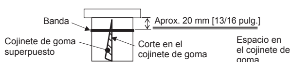
<Fig. 6: Parte posterior del cojinete de goma>
