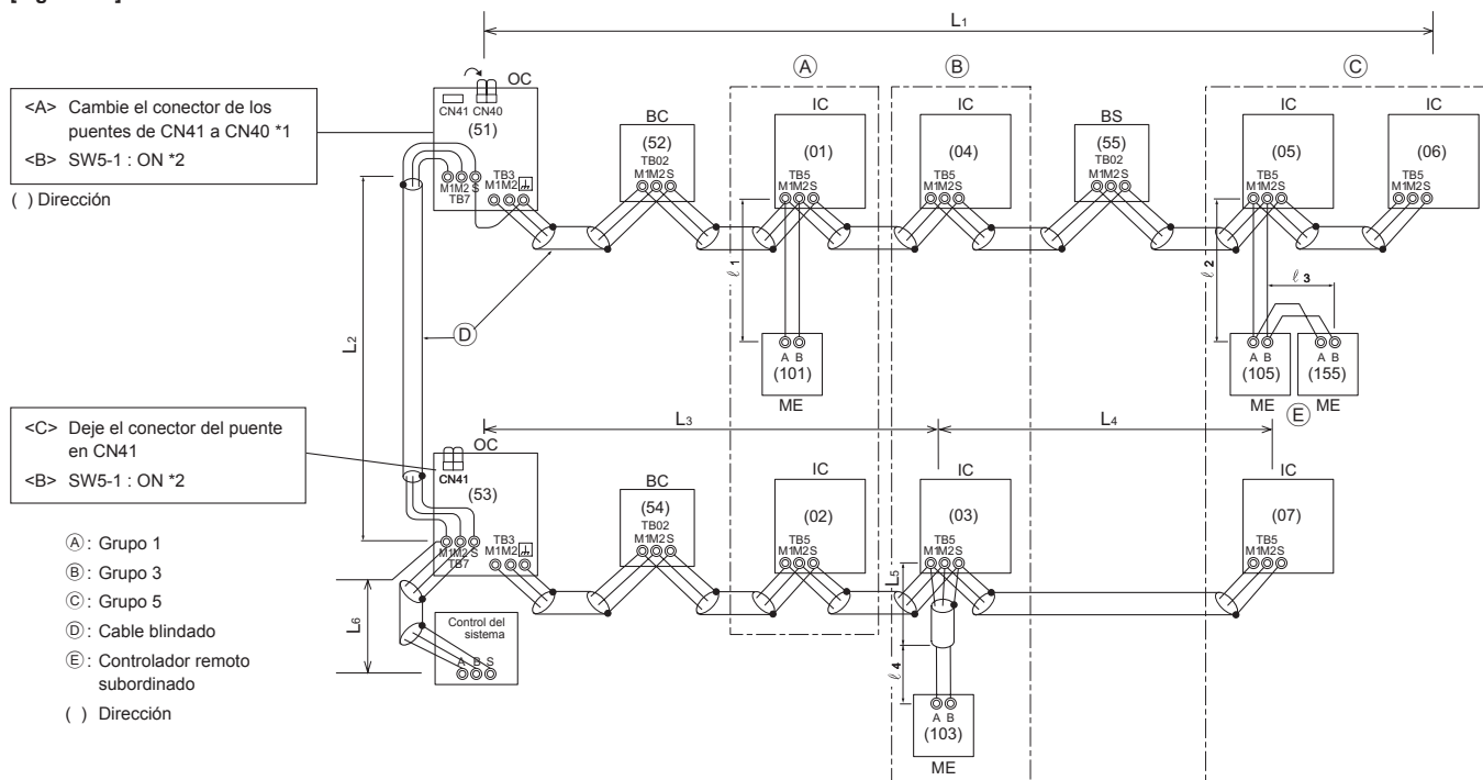
[Fig. 11.3.1] Controlador remoto M-NET
