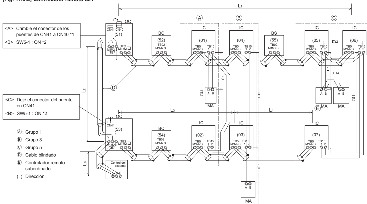
[Fig. 11.3.2] Controlador remoto MA
