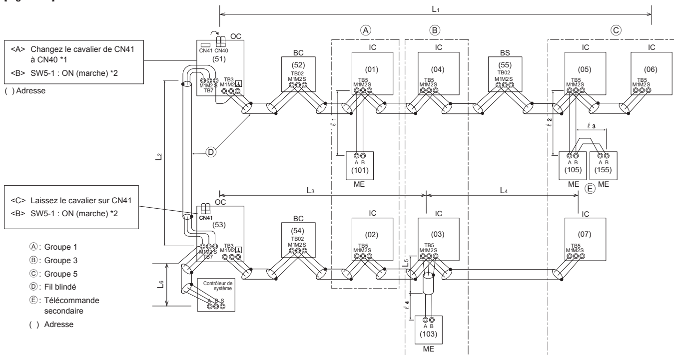
[Fig. 11.3.1] Télécommande M-NET
