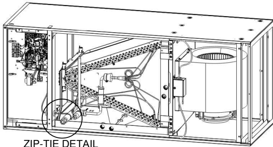
ZIP-TIE DETAIL
