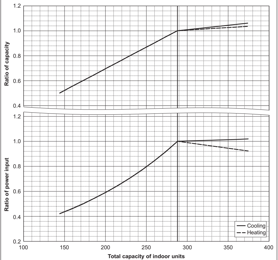
PQHY-P312TSLMU/YSLMU-A
