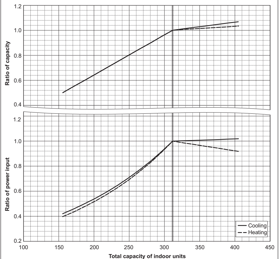
PQHY-P312TSLMU/YSLMU-A
