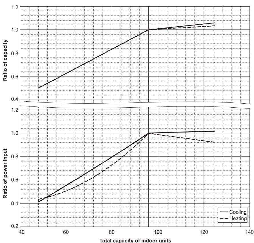
PQHY-P96TLMU/YLMU-A
