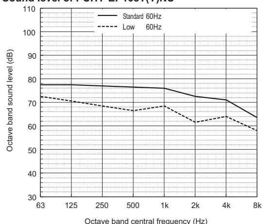
Sound level of PUHY-EP168T(Y)NU
