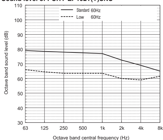
Sound level of PUHY-EP192T(Y)SNU
