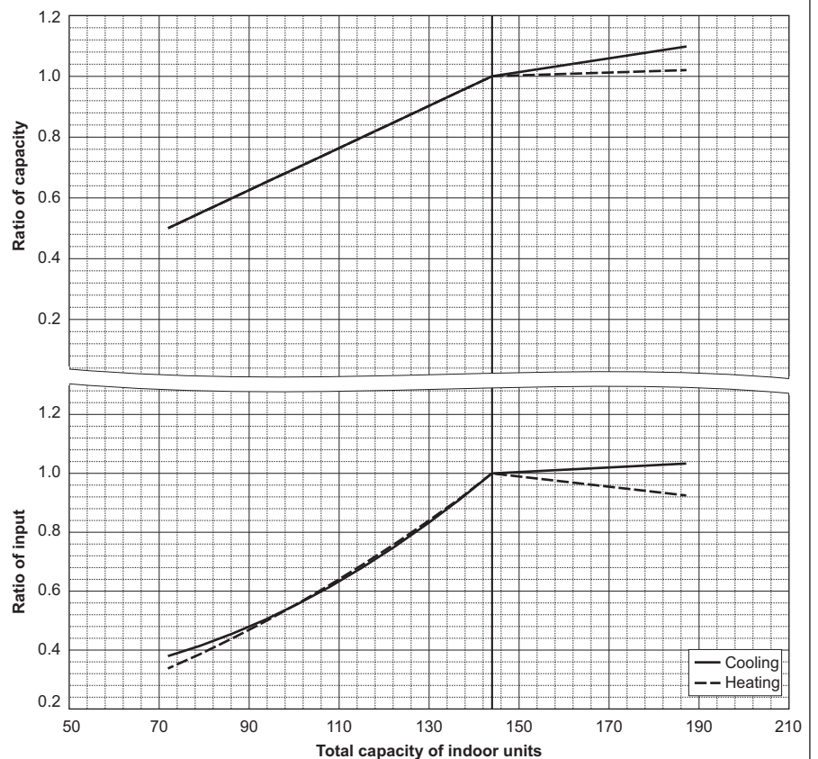
PUHY-P144TNU/YNU-A1
