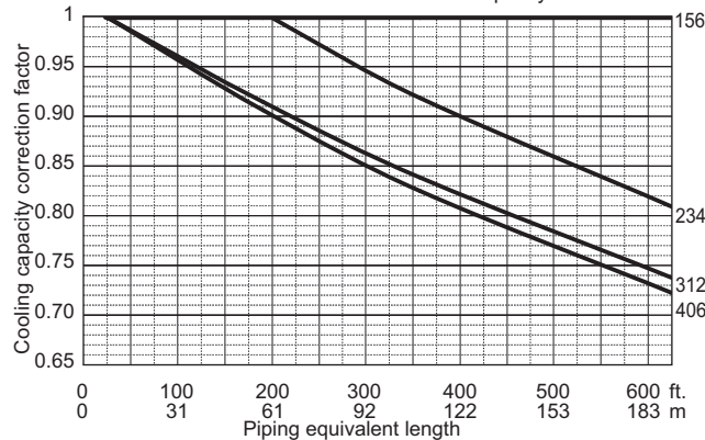
PUHY-P336TSNU/YSNU
