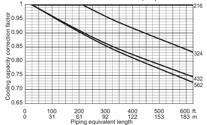
PUHY-P432TSNU/YSNU
