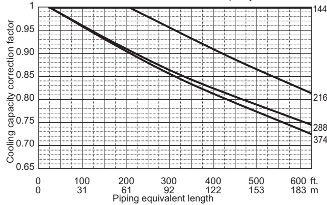
PUHY-P312TSNU/YSNU
