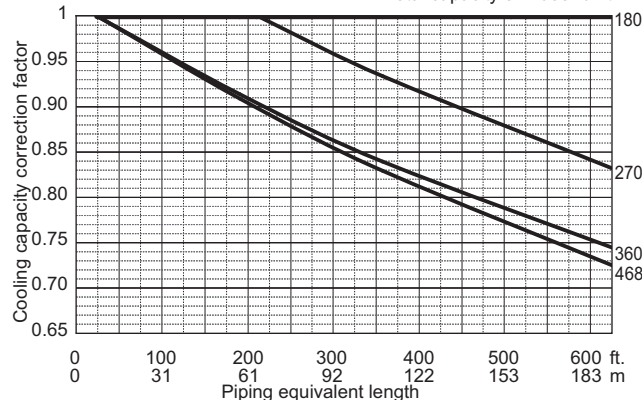
PUHY-P360TSNU/YSNU
