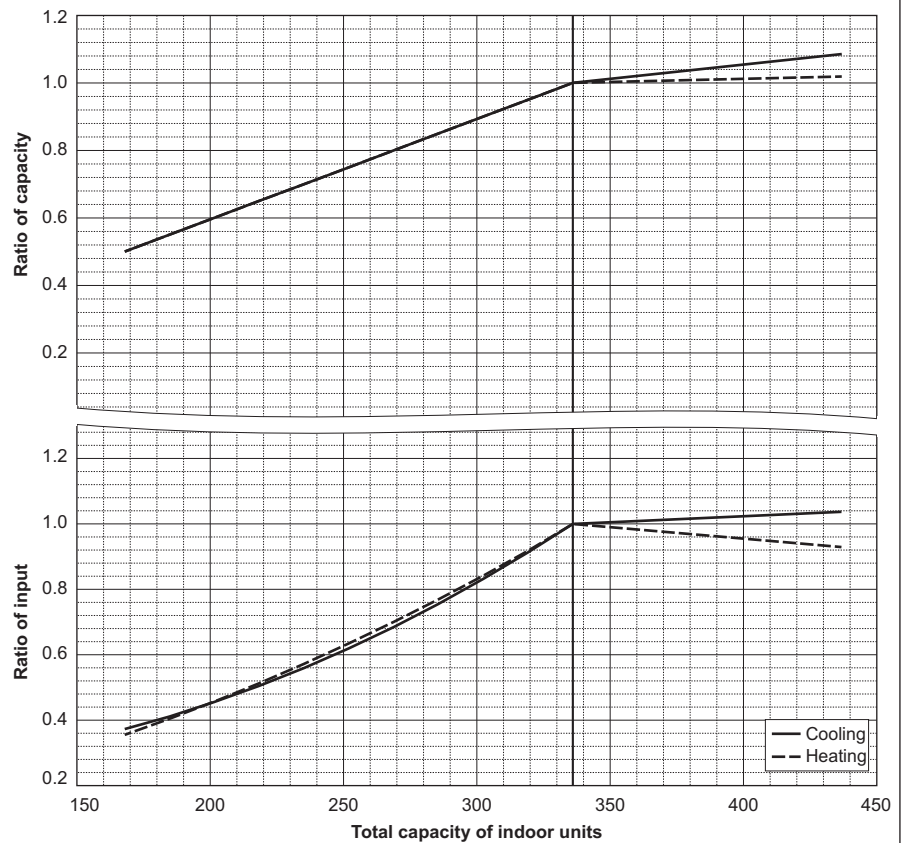
PUHY-P360TSNU/YSNU-A1
