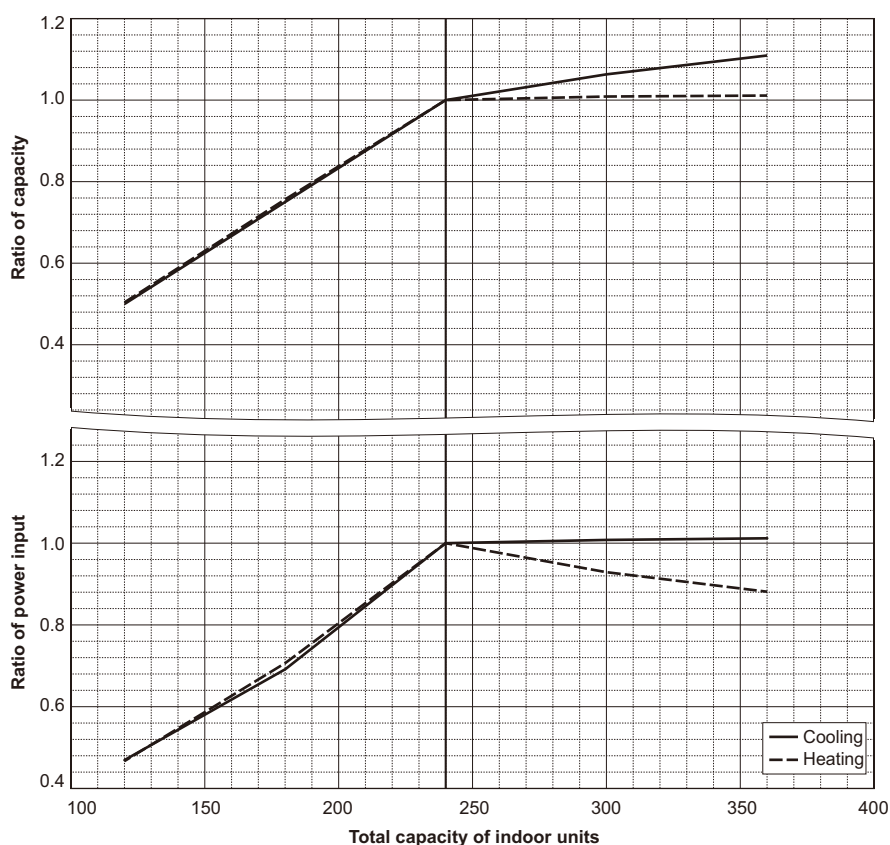
PURY-P240TSNU/YSNU-A
