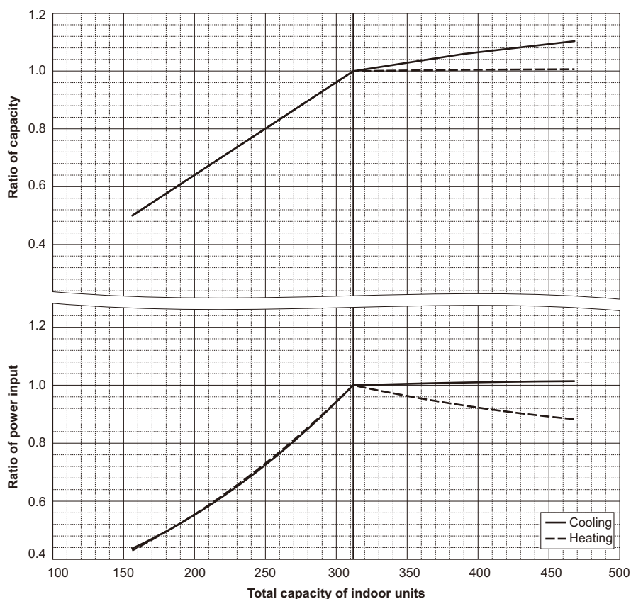
PURY-P336TSNU/YSNU-A
