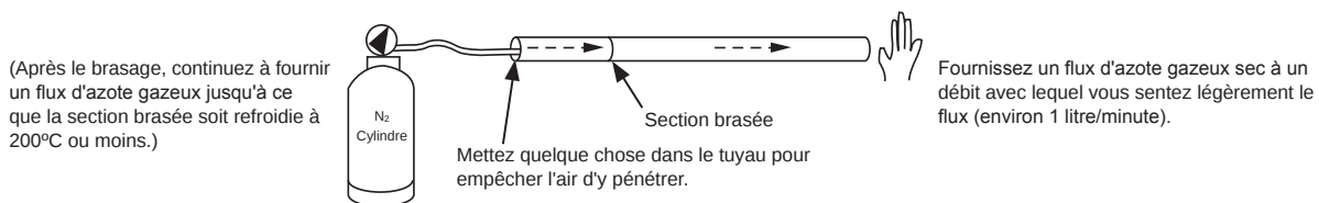
Exemple de tuyaux de brasage sous purge à l'azote
