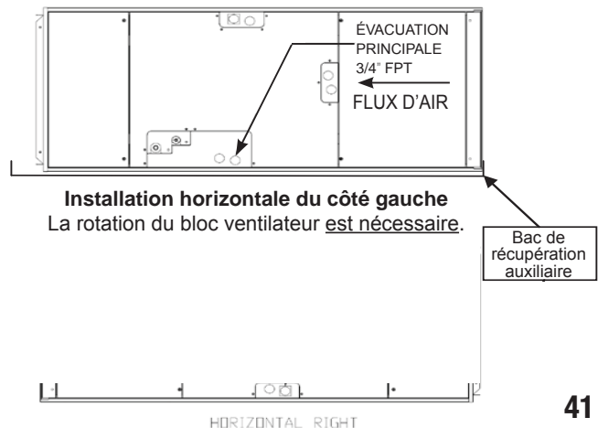
Étape 14d Ensuite, installez les tubes en plastique transparent qui sont inclus dans le sac d'accessoires. Assurez-vous que les tubes en plastique permettent l'évacuation dans le bac. Vérifiez également que les tubes en plastique transparent ne comportent aucune restriction. Il est nécessaire de couper les tubes en plastique, reportez-vous au tableau relatif à la longueur des tubes. Enfin, fixez les tubes en plastique transparent au bac de récupération supérieur comme indiqué par le Détail A, puis fixez-les aux supports métalliques de fixation de la bobine au bac de récupération supérieur à l'aide des serre-câbles en plastique fournis comme indiqué.
