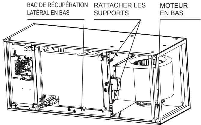
Étape 15 Réinstallez la bobine ainsi que le(s) support(s) de fixation. Ne pas réinstaller les supports entraînera une perte de capacité et la formation de condensation à l'intérieur du caisson. Le faisceau électrique pour le connecteur de la thermistance doit également être acheminé à nouveau dans la partie électrique et branché à CN44. Reportez-vous à 9.3. Étape 1 à 4 en procédant dans l'ordre inverse pour remonter les panneaux. Assurez-vous que les orifices défonçables appropriés sont retirés pour les raccords d'évacuation et les connexions électriques.
