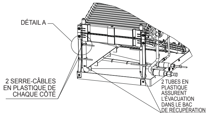
Étape 14d Ensuite, installez les tubes en plastique transparent qui sont inclus dans le sac d'accessoires. Assurez-vous que les tubes en plastique permettent l'évacuation dans le bac. Vérifiez également que les tubes en plastique transparent ne comportent aucune restriction. Il est nécessaire de couper les tubes en plastique, reportez-vous au tableau relatif à la longueur des tubes. Enfin, fixez les tubes en plastique transparent au bac de récupération supérieur comme indiqué par le Détail A, puis fixez-les aux supports métalliques de fixation de la bobine au bac de récupération supérieur à l'aide des serre-câbles en plastique fournis comme indiqué.
