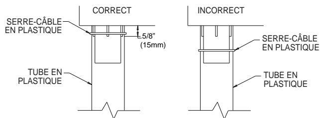
DÉTAIL A
