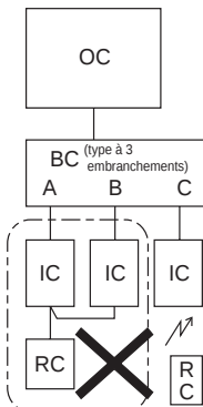
3-1. Fonctionnement groupé au moyen d'une seule télécommande
