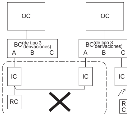
3-2. Funcionamiento agrupado entre distintos sistemas refrigerantes
