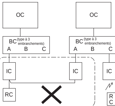
3-2. Fonctionnement groupé entre différents systèmes réfrigérants
