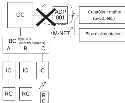
3-3. Raccordement d'un adaptateur M-NET à l'appareil extérieur
