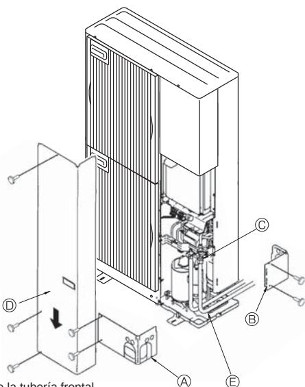
A Cubierta de la tubería frontal B Cubierta de la tubería C Válvula de parada D Panel de servicio E Radio del codo: 100 mm - 150 mm [3-15/16" - 5-7/8"]
