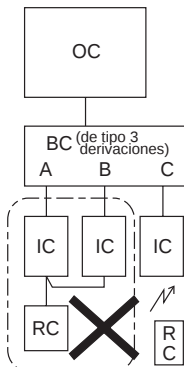
3-1. Funcionamiento agrupado mediante un único controlador remoto
