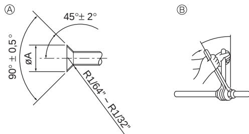
A Dimension de l'évasement B Couple de serrage du raccord conique
