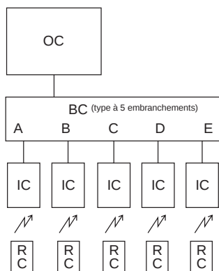
2-2. Type à 5 embranchements uniquement
