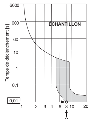
Diagramme d'échantillon du courant de déclenchement nominal (x)
