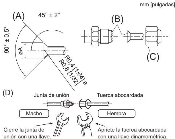
(A) Dimensiones de corte abocardado (D) Par de apriete de la tuerca abocardada
