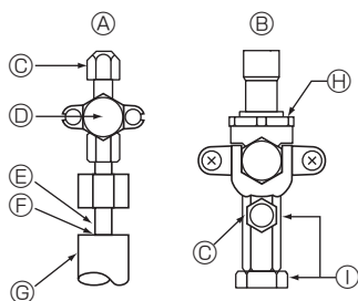
(A) Válvula de retención <Lado de líquido> (B) Válvula de retención <Lado de gas> (C) Puerto de servicio (D) Sección Abierto/Cerrado (E) Tubo local (F) Sellado, igual para lado de gas (G) Cubierta del tubo (H) No utilice una llave aquí. Podría producirse una pérdida de refrigerante. (I) Utilice 2 llaves aquí.
