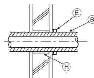
(6) Protección de las piezas penetrantes en paredes antiincendio y divisorias
