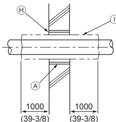
(6) Protección de las piezas penetrantes en paredes antiincendio y divisorias
