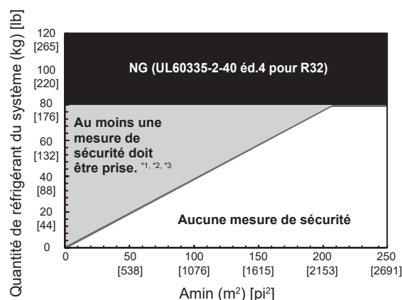
Fig. 1 Concentration de réfrigérant et mesure de sécurité requise (hauteur du plafond = 2,5 m [8-3/16 pi])
