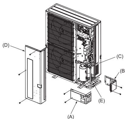
(A) Couvercle de la tuyauterie avant (B) Couvercle de la tuyauterie (C) Vanne d'arrêt (D) Panneau de service (E) Rayon de cintrage : 100 mm, 3-15/16 pouces-150 mm, 5-27/32 pouces
