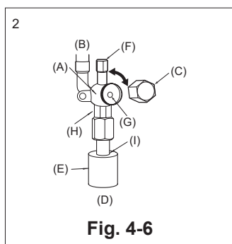
(A) Corps de vanne (B) Côté appareil (C) Capuchon (D) Côté tuyau local (E) Gaine du tuyau (F) Orifice pour l'entretien (G) Tige de vanne (H) Côté clé double (I) Côté joint d'étanchéité (Utiliser une clé de ce côté uniquement. Dans le cas contraire, une fuite de liquide pourrait en résulter.) (Etancher l'extrémité de l'isolation thermique du côté du raccord du tuyau avec un produit d'étanchéité quelconque pour éviter toute infiltration d'eau dans le matériel d'isolation thermique.)
