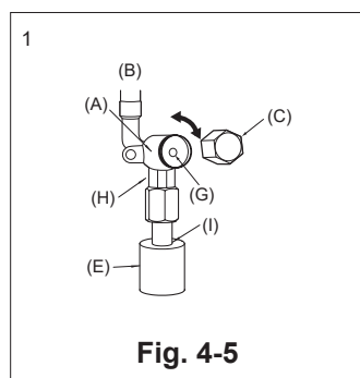
(A) Corps de vanne (B) Côté appareil (C) Capuchon (D) Côté tuyau local (E) Gaine du tuyau (F) Orifice pour l'entretien (G) Tige de vanne (H) Côté clé double (Utiliser une clé de ce côté uniquement. Dans le cas contraire, une fuite de liquide pourrait en résulter.) (I) Côté joint d'étanchéité (Etancher l'extrémité de l'isolation thermique du côté du raccord du tuyau avec un produit d'étanchéité quelconque pour éviter toute infiltration d'eau dans le matériel d'isolation thermique.)
