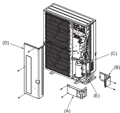
(A) Couvercle de la tuyauterie avant (B) Couvercle de la tuyauterie arrière (C) Vanne d'arrêt (D) Panneau de service (E) Rayon de cintrage : 100 mm, 3-15/16 pouces-150 mm, 5-27/32 pouces
