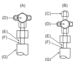
(A) Vanne d'arrêt <côté gaz> (B) Vanne d'arrêt <côté liquide> (C) Orifice pour l'entretien (D) Section d'ouverture/fermeture (E) Tuyau local (F) Hermétique, idem pour le côté gaz (G) Fourrure du tuyau (H) Ne pas utiliser de clé ici. (I) Utiliser deux clés ici.
