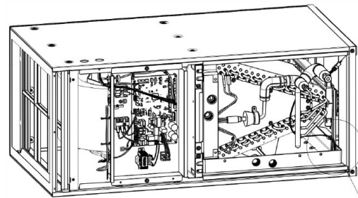
ZIP-TIE DETAIL
