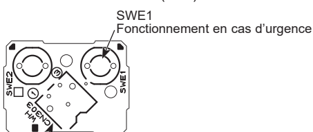
CN303 Carte contrôleur intérieure (I.B.) Connecté au CNRU
