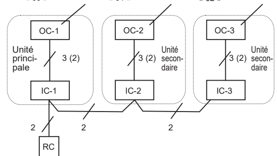
Fig. 1 Adresse du réfrigérant « 00 » Adresse du réfrigérant « 01 » Adresse du réfrigérant « 02 »
