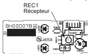
CN301 Carte contrôleur intérieure (I.B.) Connecté au CNRU
