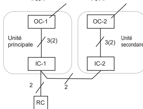
Fig. 1 Adresse du réfrigérant « 00 » Adresse du réfrigérant « 01 »
