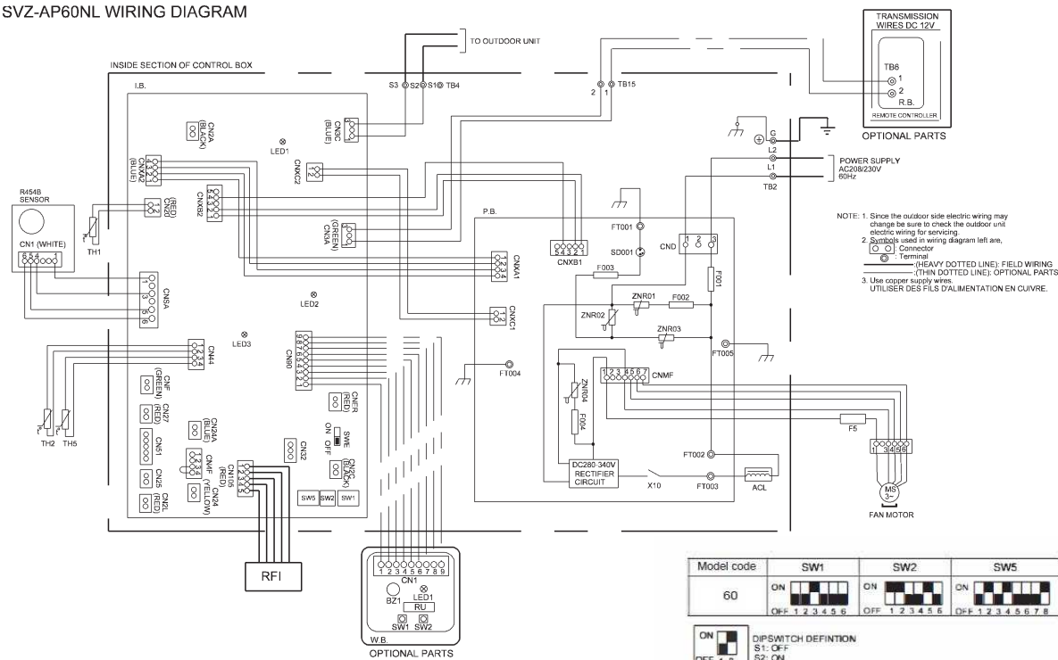
SVZ-AP60NL WIRING DIAGRAM
